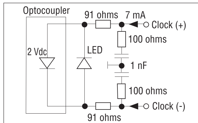
Fig. 10: Sensor input
