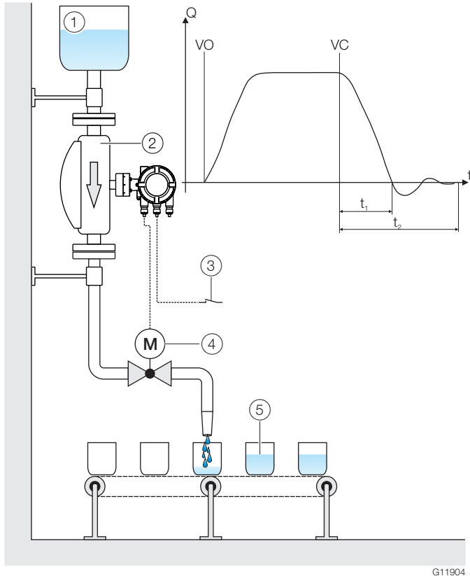
Fig. 3: FillMass fill function ① Collection tank ② Sensor ③ Fill start / stop (digital input via plug-in card) ④ Fill valve ⑤ Fill container
